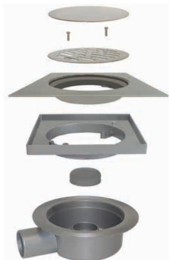
Esploso dei componenti
