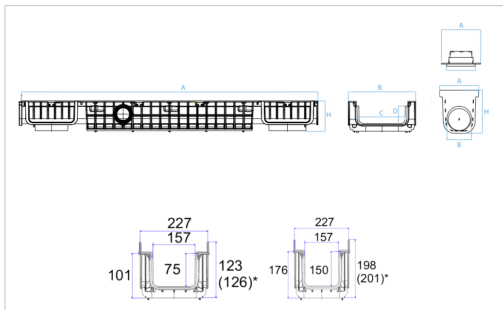
Scarichi laterali H 7,5: scarico Ø 50 - 63 H15: Scarico Ø 80 - 100 - 110
