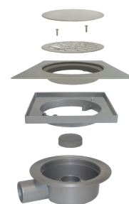
ESPLOSO
