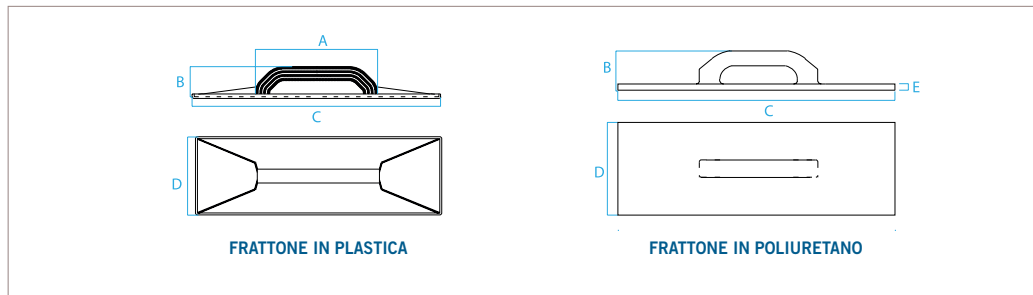
Piano levigatore del frattone in poliuretano espanso
