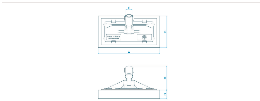
Dettaglio dell'aggancio del manico
